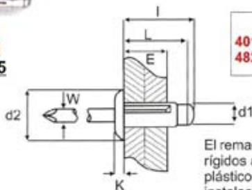
Cabeza aluminio Al Mg 2.5 Vástago aluminio Al Mg 2.5
