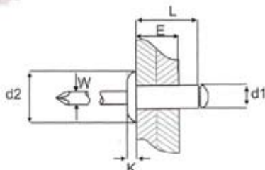
Cabeza aluminio Al Mg 3.5 Vástago en acero cincado
